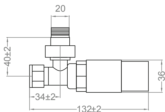
valve avec tête thermostatique
