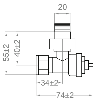
valve thermostatique
