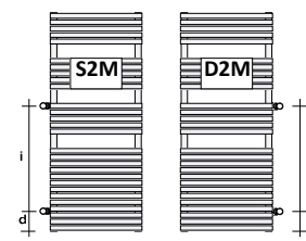
Spécifier « i » et « d » i min.=5 cm d min.=2 cm
