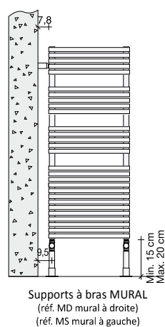
Support STANDARD MURAL (réf. ST)
